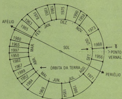
Fig. 4 - Órbitas de Marte e da Terra com as oposições de 1954 a 1999. As órbitas aparecem circulares em primeira aproximação.
