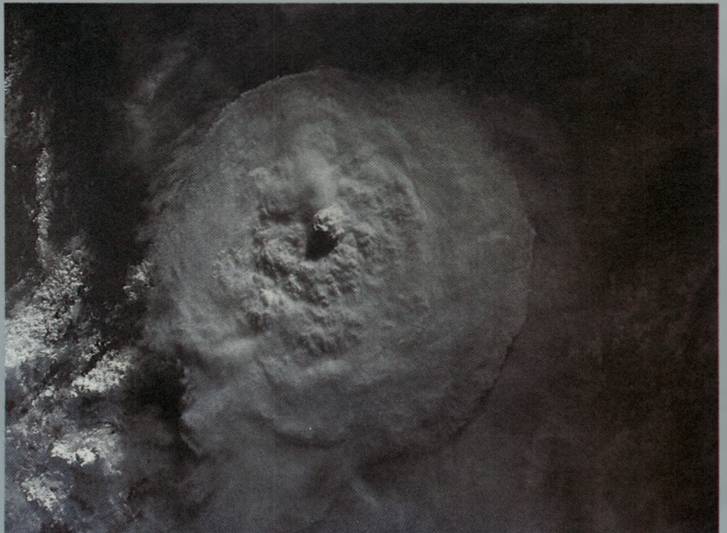
Fig 8 – O monte Olimpo, o maior vulcão conhecido do sistema solar. A largura de sua lava equivale a distância aproximadamente entre Rio e São Paulo. Sua altura é o equivalente a um prédio, imaginário, de 6666 andares.
