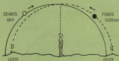
Fig. 5 - Cruzamento aparente de Fobos e Deimos para um observador em Marte
